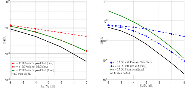
그림 2 적응형 수신 빔포밍 기술의 BER 성능
